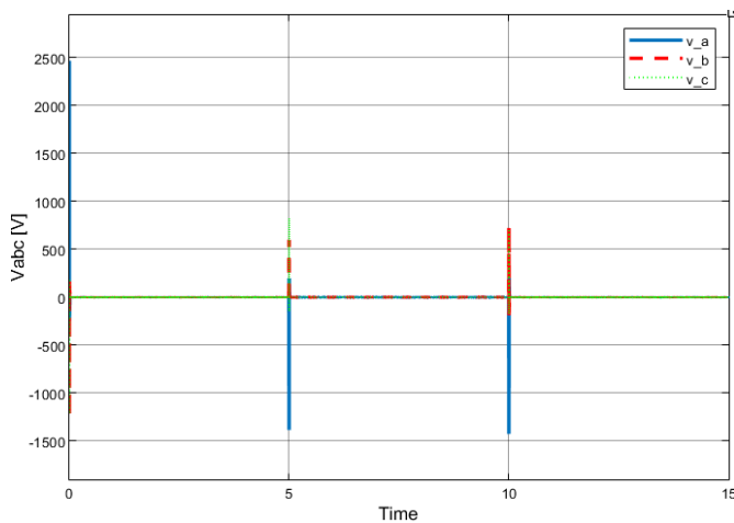
Figura 47: Tensiones v_{abc}(t)
